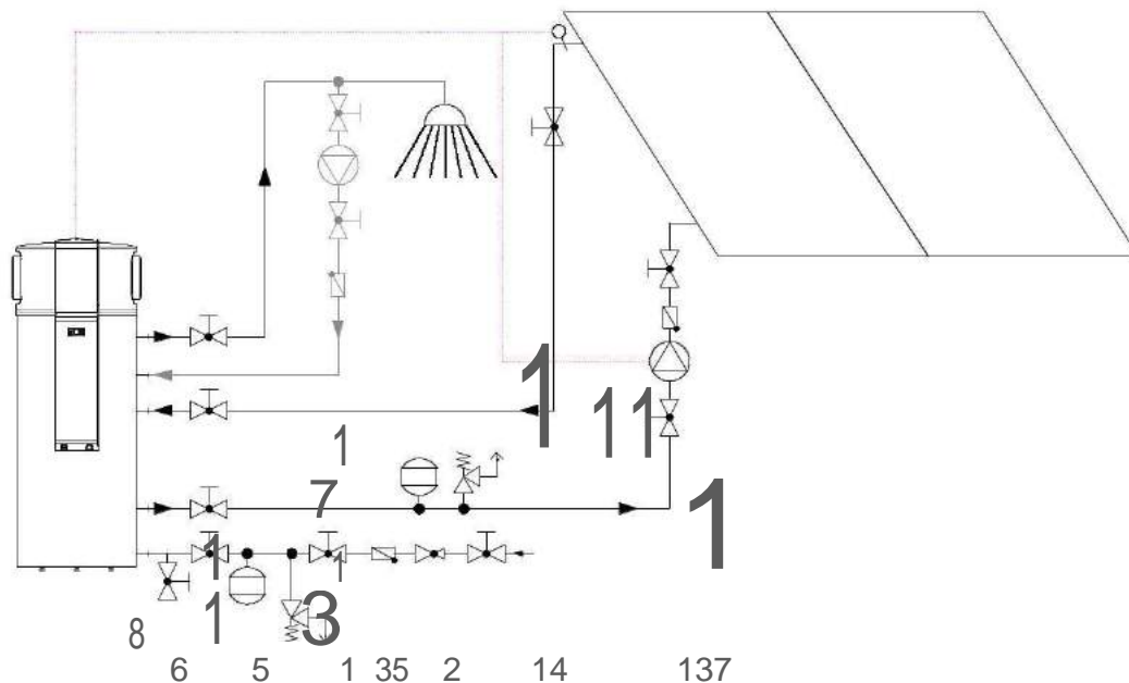
Abbildung 4: Wärmepumpe in Kombination mit Solarkollektoren
