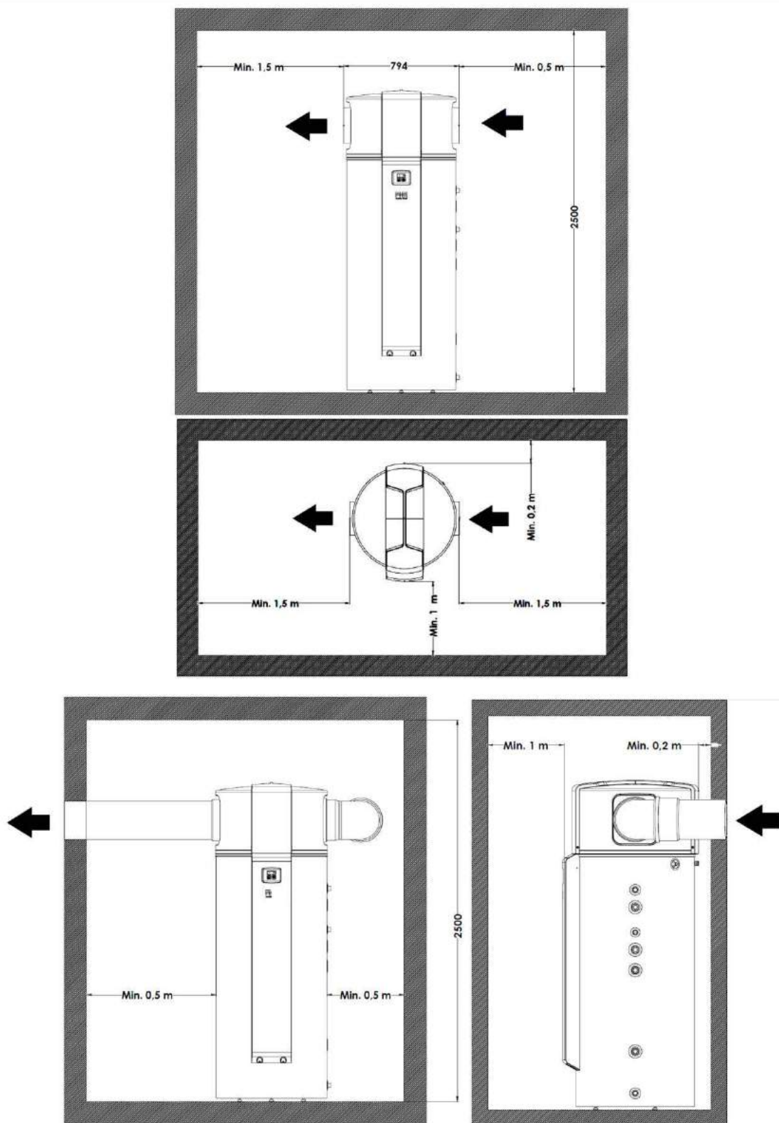
Mindestabstände für den Luftdurchlass
