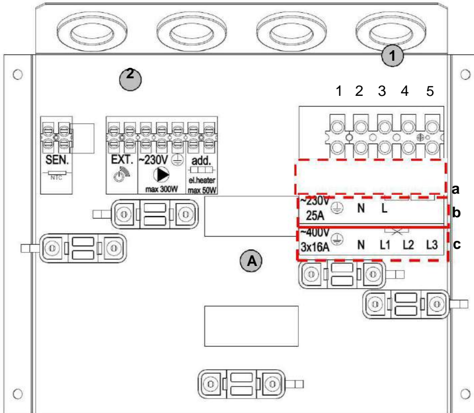
Abbildung 7: Elektrische Anschlüsse
